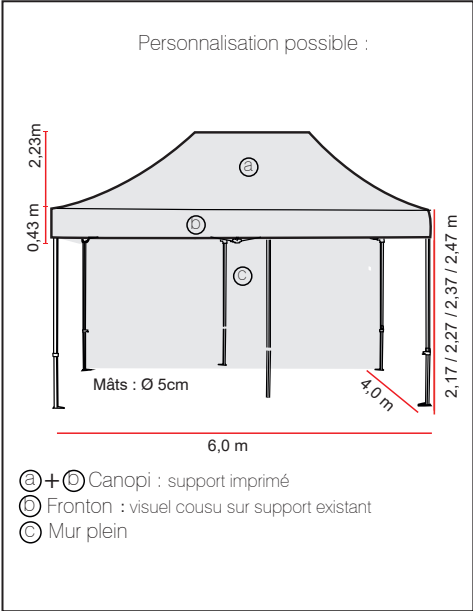
Dimensions produit
